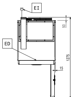
Boven aanzicht
